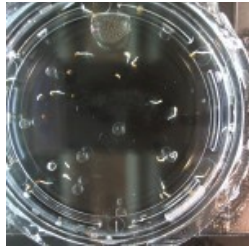
10% D2O
