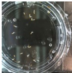
25% D2O
